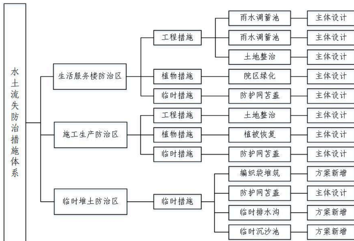
图5-1 项目水土流失防治措施体系图
